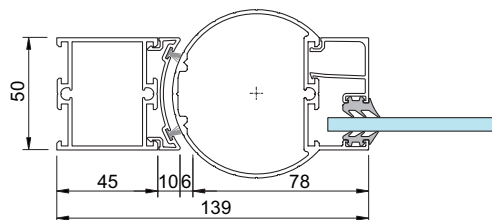
1 - Dörr med klämfri bakkant, rundad aluminiumprofil
