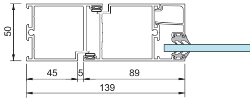
1, 2 - Dörr med smalprofil
